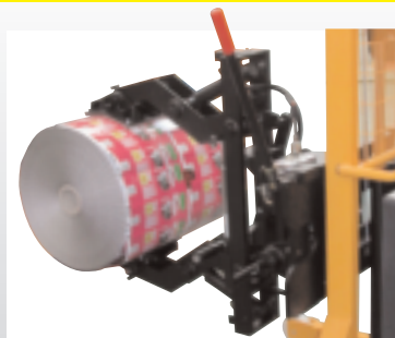
Roll Rotator
